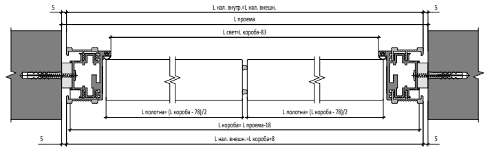
Открытие OUT Двустворчатая Дверь | OUT Opening
