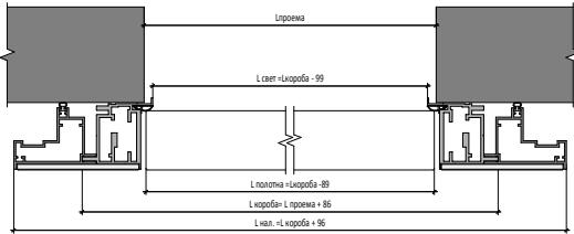
Открытие IN Двустворчатая Дверь | IN Opening
