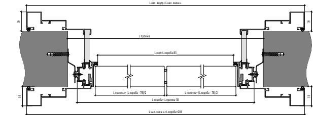
Открытие OUT Двухстворчатая Дверь | OUT Opening
