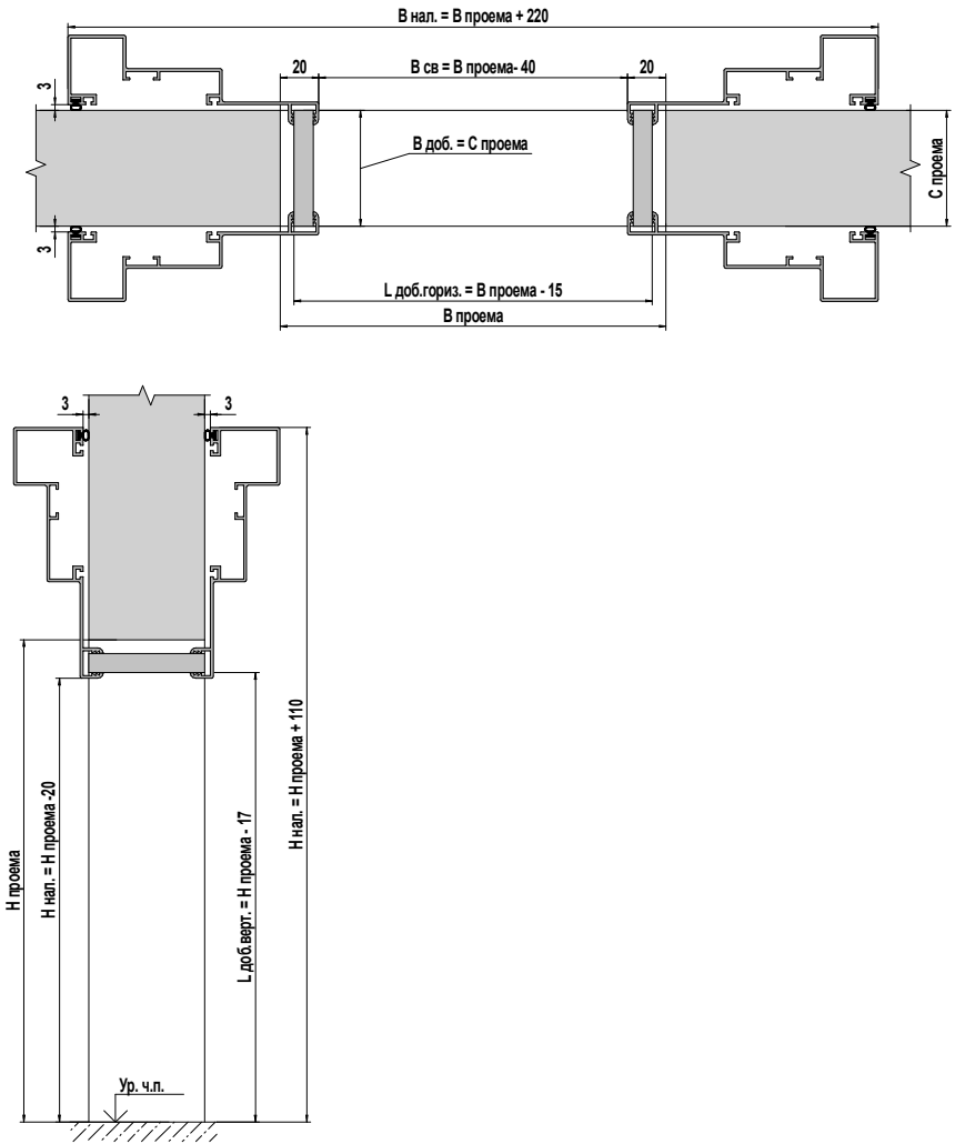
Короб Standard, наличник TRIANGOLO Standard jamb, TRIANGOLO platband
