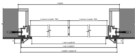
Открытие IN Двухстворчатая Дверь | IN Opening
