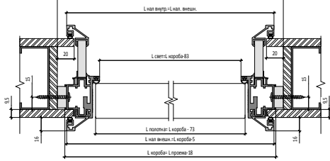
Открытие OUT Двухстворчатая Дверь | OUT Opening
