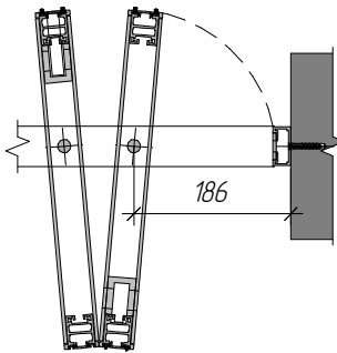
Дверь гармошка с накладным притворным профилем Folding door with laid on side runner profile
