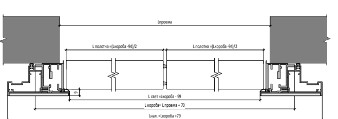
Открытие OUT Двустворчатая Дверь | OUT Opening
