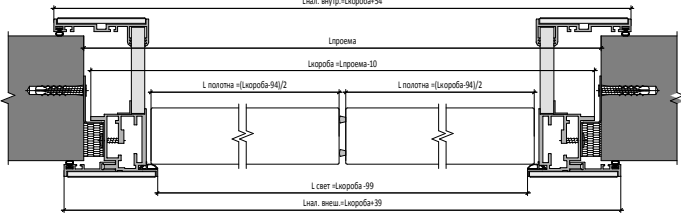
Открытие IN Двустворчатая Дверь | IN Opening
