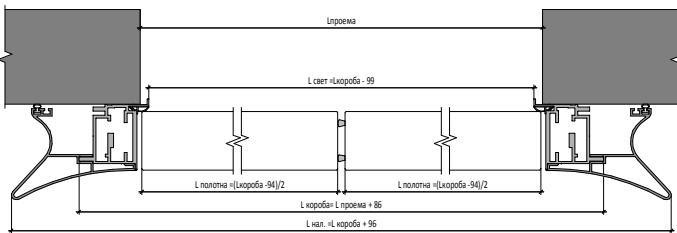
Открытие IN Двустворчатая Дверь | IN Opening
