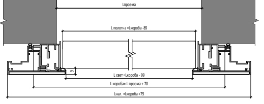
Открытие OUT Двустворчатая Дверь | OUT Opening
