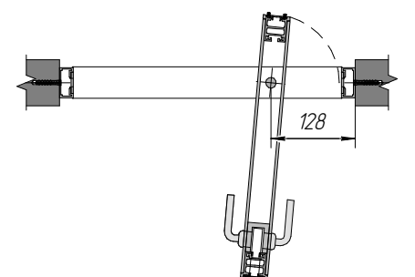
Роторная дверь с открыванием в две стороны накладным притворным профилем Bidirectional door with laid on side runner profile
