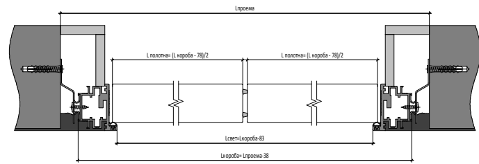
Открытие IN Двустворчатая Дверь | IN Opening
