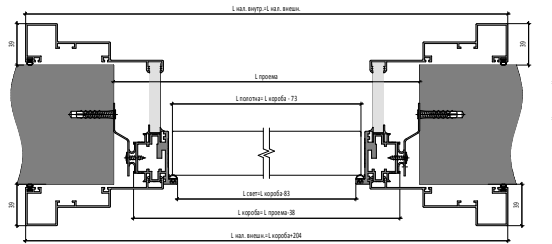
Открытие IN Двухстворчатая Дверь | IN Opening
