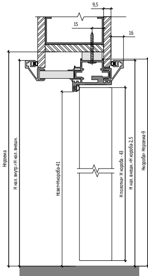
Открытие OUT | OUT Opening
