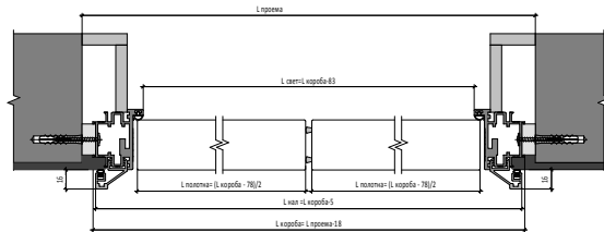
Открытие OUT Двухстворчатая Дверь | OUT Opening
