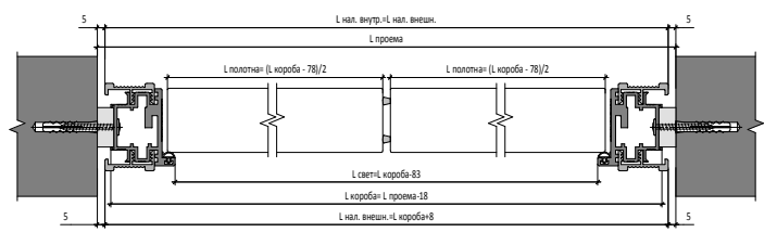
Открытие IN Двустворчатая Дверь | IN Opening
