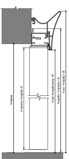
Открытие OUT | OUT Opening
