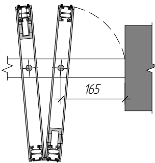
Дверь гармошка Folding door
