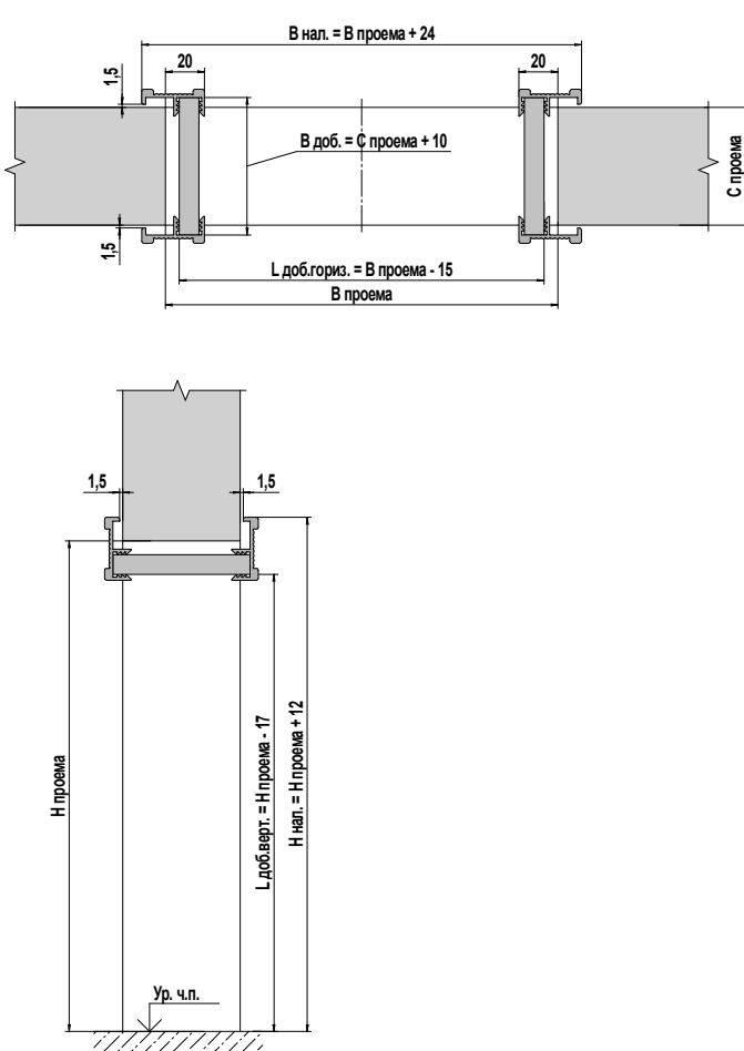
Короб Standard, наличник MINI Standard jamb, MINI platband
