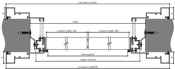
Открытие IN Двухстворчатая Дверь | IN Opening
