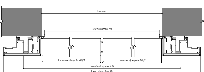
Открытие IN Двустворчатая Дверь | IN Opening
