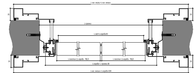
Открытие OUT Двухстворчатая Дверь | OUT Opening
