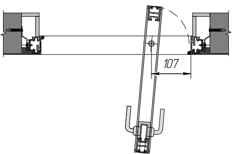
Роторная дверь с открыванием в одну сторону со стандартной дверной коробкой Bidirectional door with standard jamb
