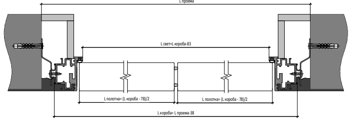
Открытие OUT Двустворчатая Дверь | OUT Opening
