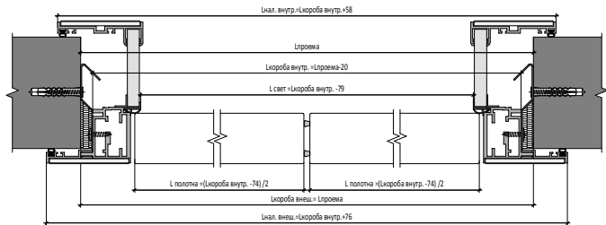
Открытие OUT Двустворчатая Дверь | OUT Opening
