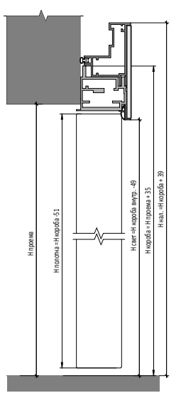
Открытие OUT | OUT Opening
