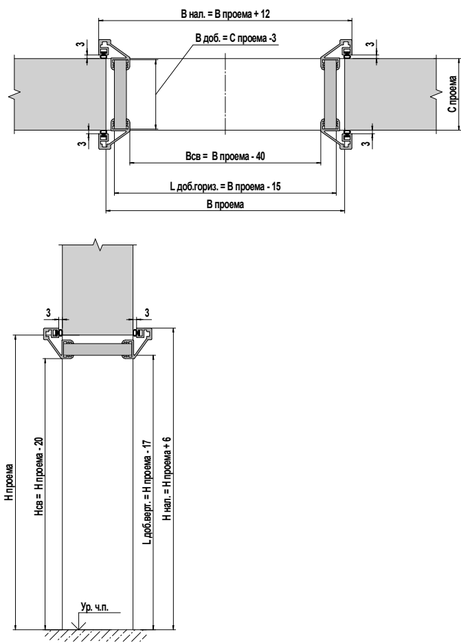
Короб Standard, наличник PASSO Standard jamb, PASSO platband
