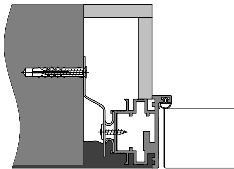
Открытие OUT | OUT Opening
