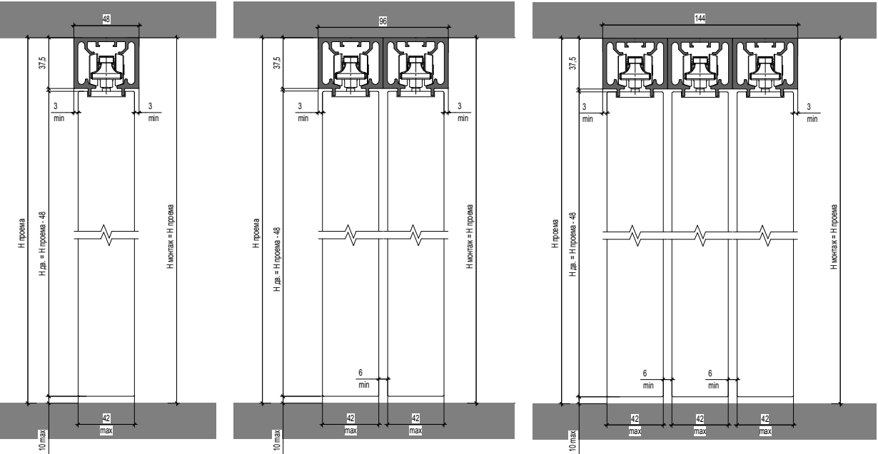
Раздвижная дверь, алюминиевый профиль, скрытое крепление Sliding door, aluminum profile, hidden mounting
