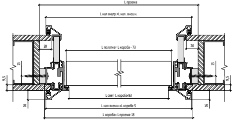
Открытие IN Двухстворчатая Дверь | IN Opening
