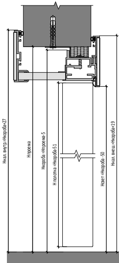
Открытие IN Двустворчатая Дверь | IN Opening
