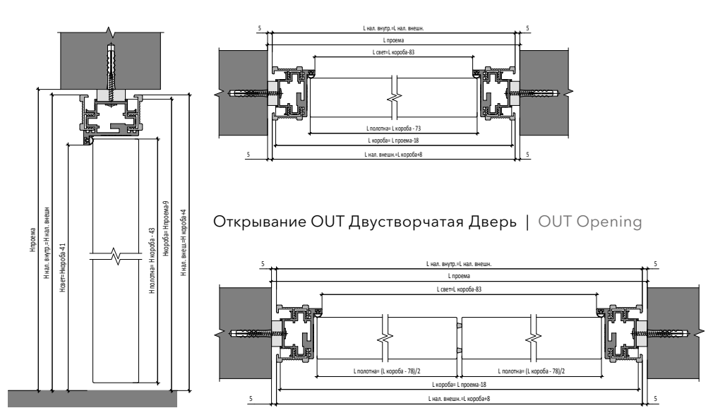
Открытие OUT | OUT Opening
