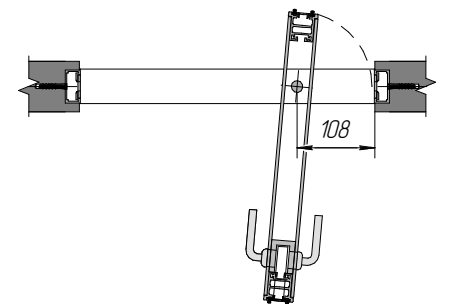
Роторная дверь с открыванием в две стороны со скрытым притворным профилем Bidirectional door with hidden side runner profile
