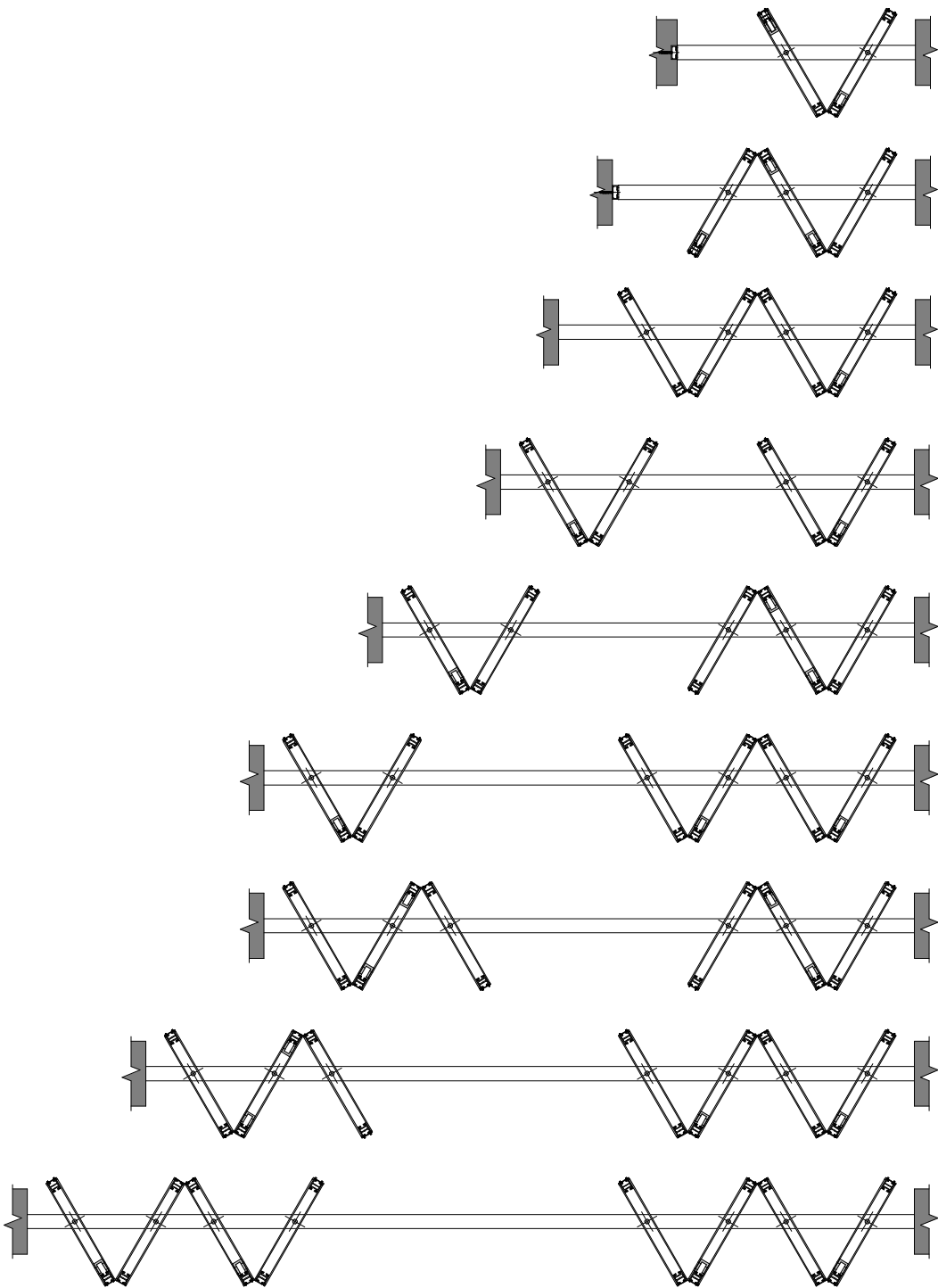
Дверь гармошка со скрытым притворным профилем Folding door with hidden side runner profile
