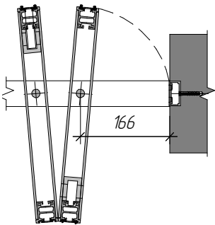
Дверь гармошка со скрытым притворным профилем Folding door with hidden side runner profile
