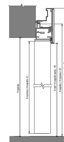
Открытие OUT | OUT Opening
