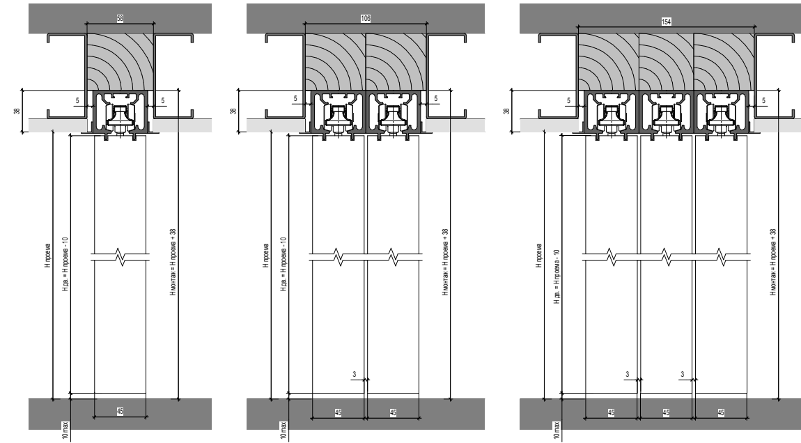
Раздвижная дверь в пенал с притворным профилем Sliding pocket door into the side runner profile
