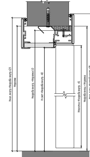
Открытие OUT Двустворчатая Дверь | OUT Opening
