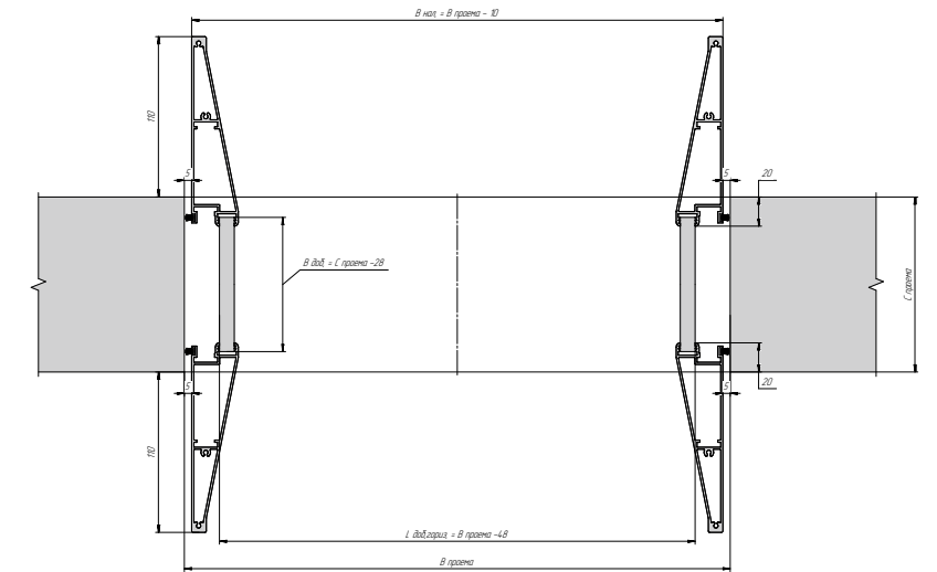
Короб Standard, наличник PORTALE Standard jamb, PORTALE platband
