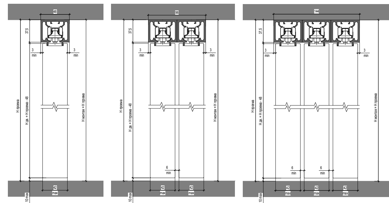
Раздвижная дверь, алюминиевый профиль, крепление в потолок Sliding door, aluminum profile, ceiling mounting
