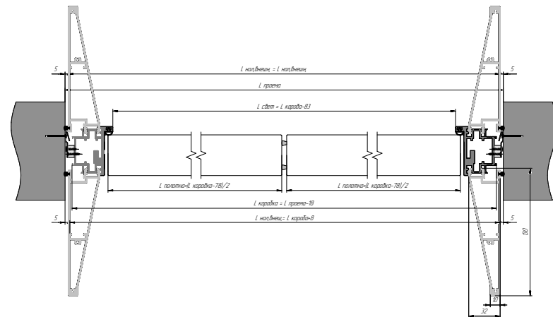
Открытие IN Двустворчатая Дверь | IN Opening
