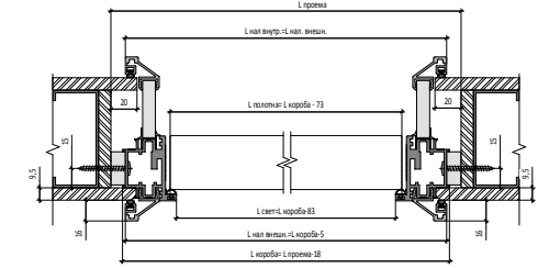
Открытие IN Двустворчатая Дверь | IN Opening
