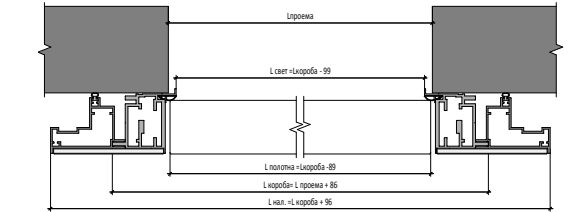
Открытие IN Двухстворчатая Дверь | IN Opening
