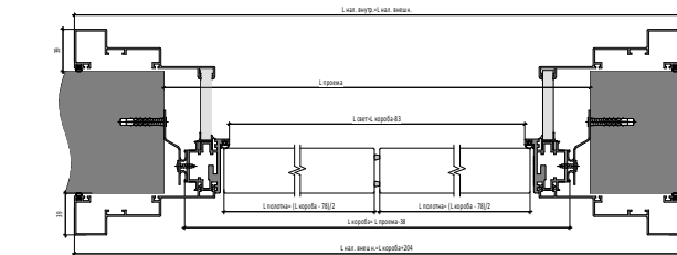
Открытие OUT Двустворчатая Дверь | OUT Opening
