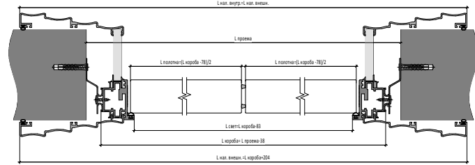
Размеры двери по ширине (L) для стандартных проёмов IN/OUT для двустворчатых дверей с наличниками CASCADE и DUNE
