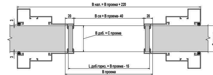
Короб Standard, наличник TRIANGOLO Standard jamb, TRIANGOLO platband
