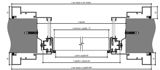
Открытие IN Двустворчатая Дверь | IN Opening
