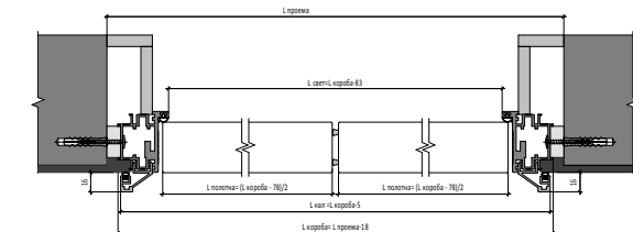
Открытие OUT Двустворчатая Дверь | OUT Opening
