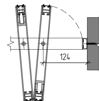
Дверь гармошка с накладным притворным профилем Folding door with laid on side runner profile
