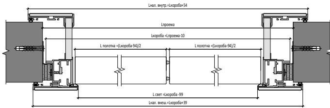
Открытие IN Двустворчатая Дверь | IN Opening
