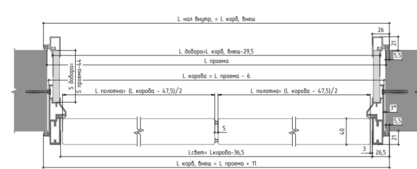
Открытие OUT Двустворчатая Дверь | OUT Opening
