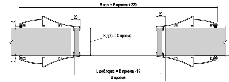
Короб Standard, наличник DUNE Standard jamb, DUNE platband
