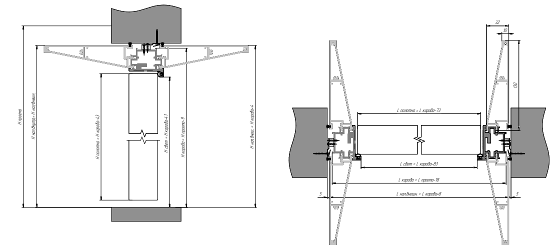
Открытие OUT Двустворчатая Дверь | OUT Opening
