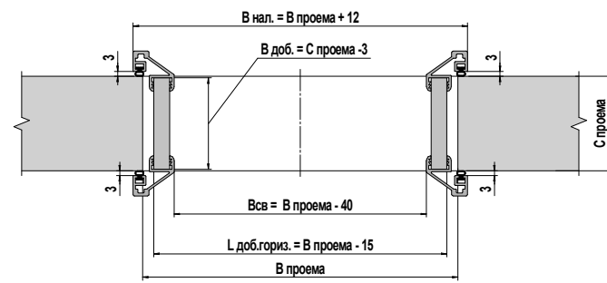
Короб Standard, наличник PASSO Standard jamb, PASSO platband
