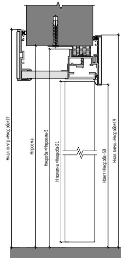
Открытие IN Двустворчатая Дверь | IN Opening
