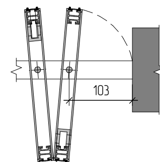
Дверь гармошка Folding door
