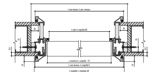
Открытие OUT Двустворчатая Дверь | OUT Opening
