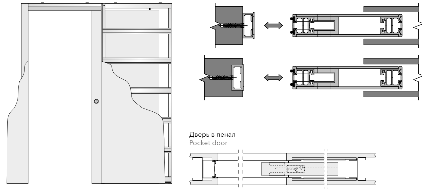
Раздвижная дверь в пенал с притворным профилем Sliding pocket door into the side runner profile
