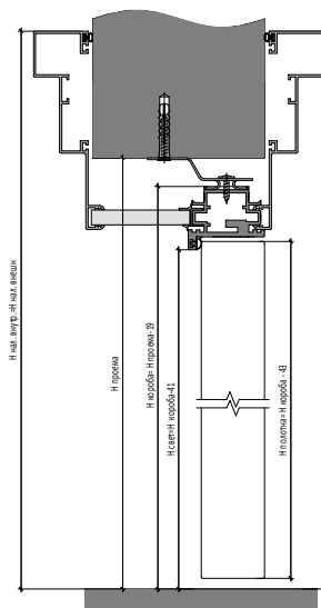
Открытие OUT | OUT Opening
