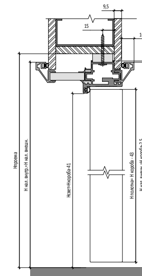
Открытие OUT | OUT Opening
