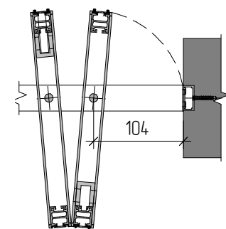
Дверь гармошка со скрытым притворным профилем Folding door with hidden side runner profile
