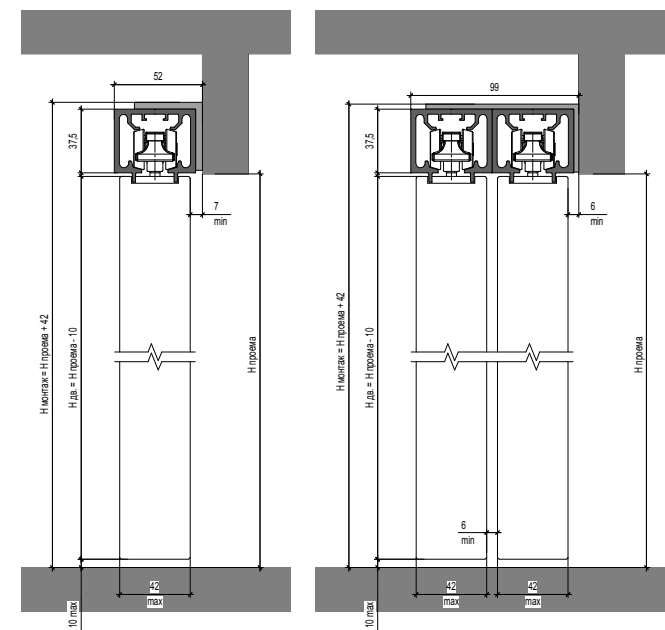
Раздвижная дверь, алюминиевый профиль, крепление к стене Sliding door, aluminum profile, wall mounting
