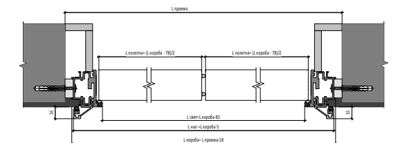
Открытие IN Двустворчатая Дверь | IN Opening
