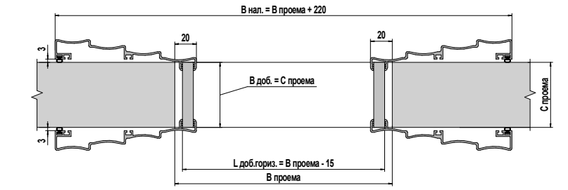
Короб Standard, наличник CASCADE Standard jamb, CASCADE platband
