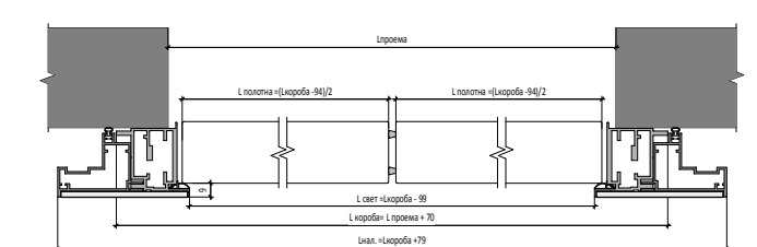
Открытие OUT Двухстворчатая Дверь | OUT Opening
