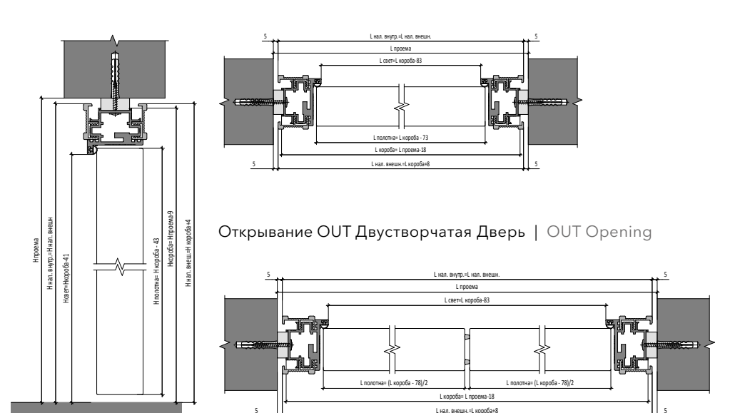
Открытие OUT | OUT Opening
