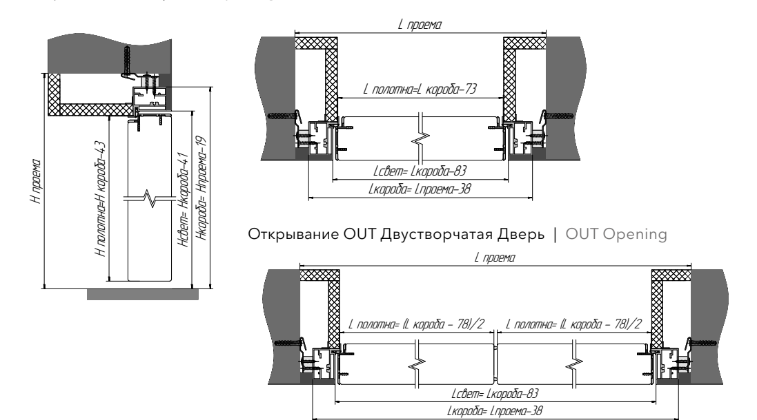
Открытие OUT | OUT Opening
