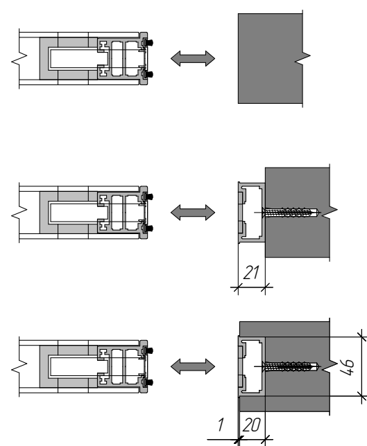
Стандартное примыкание Standard junction
