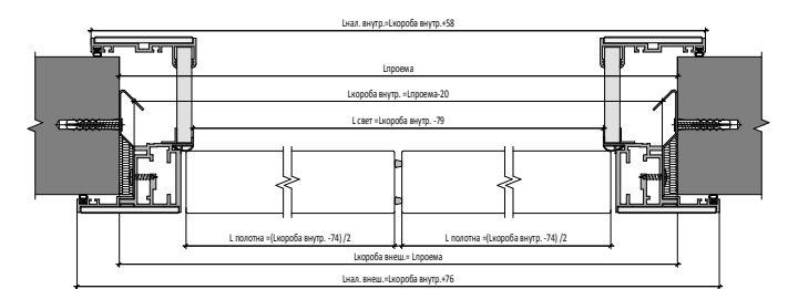
Открытие OUT Двустворчатая Дверь | OUT Opening
