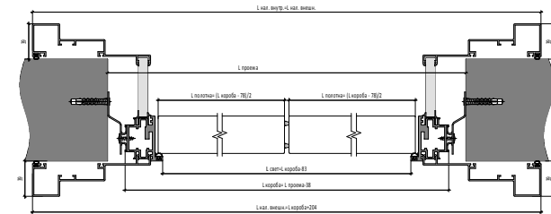
Открытие IN Двустворчатая Дверь | IN Opening
