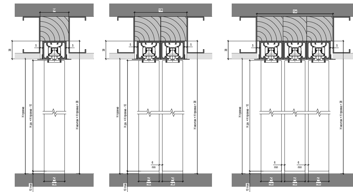
Раздвижная дверь, алюминиевый профиль, скрытое крепление Sliding door, aluminum profile, hidden mounting
