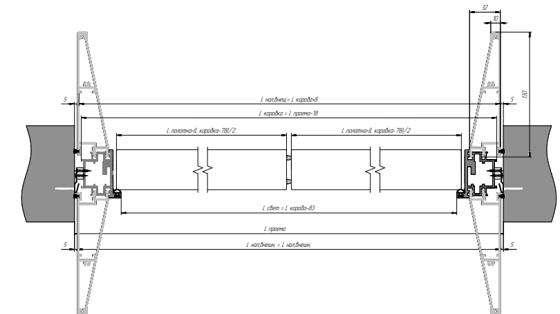
Открытие OUT Двустворчатая Дверь | OUT Opening
